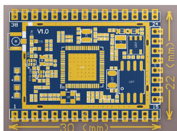
图 1 HLK-RM58S 封装大小
