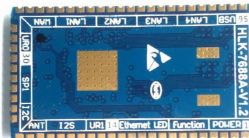
HLK-7688A 背面图
