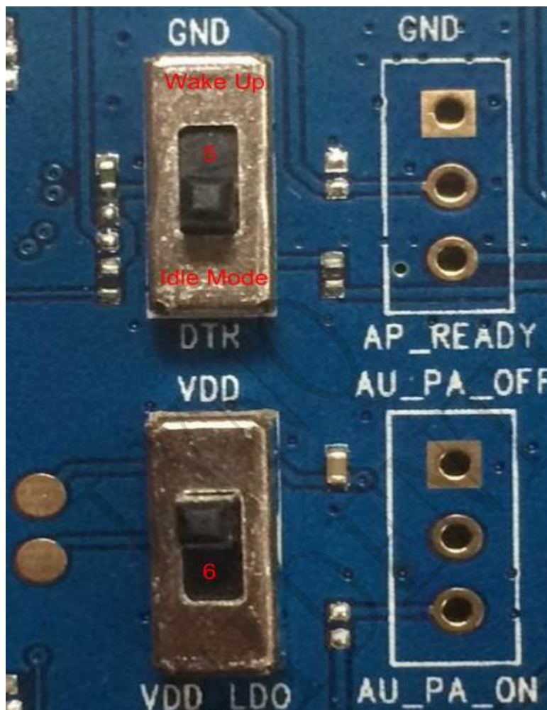
图 2-6 DTR 开关
