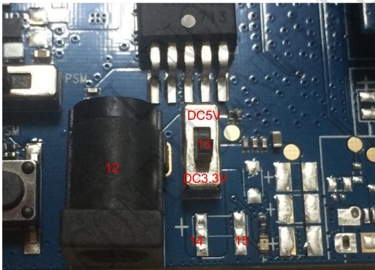
图 2-1 L620 开发板供电及开关
