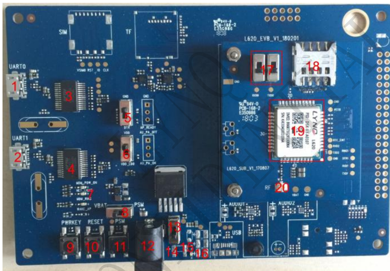
图 1-1 L620 开发板 TOP 面
