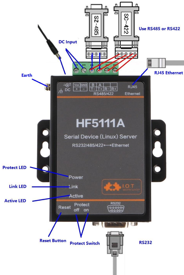
Figure 2. HF5111A 正面图
