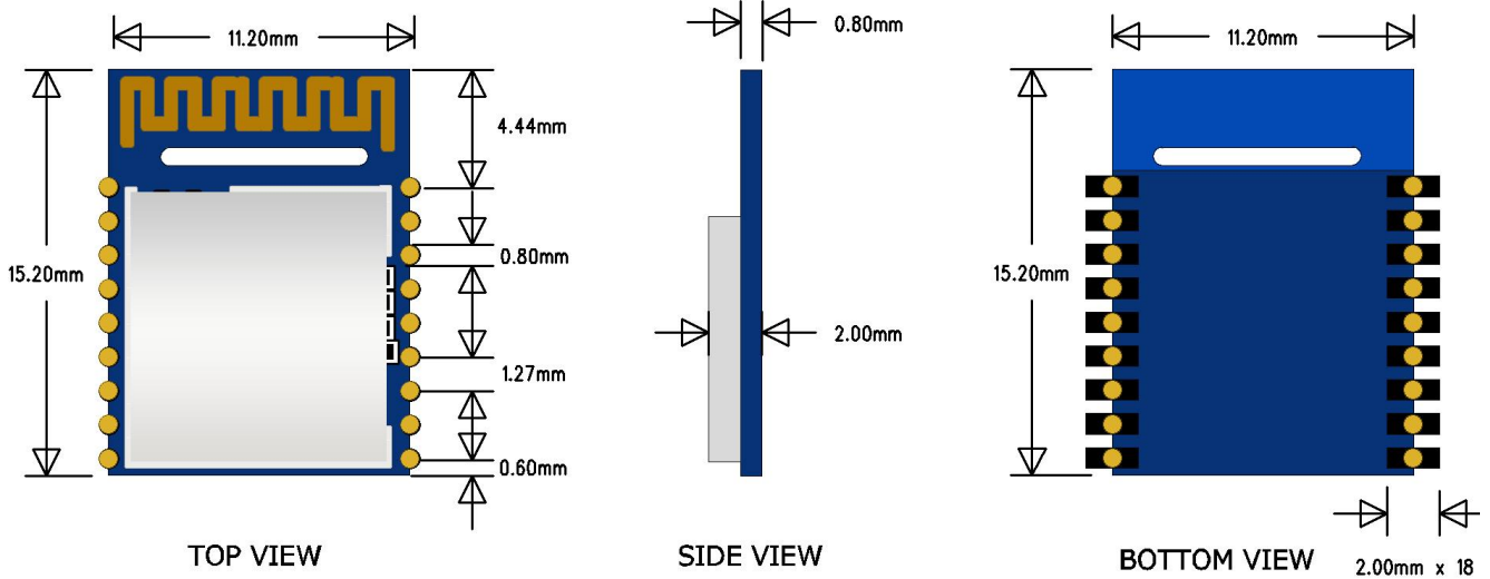
图2 模块尺寸图
