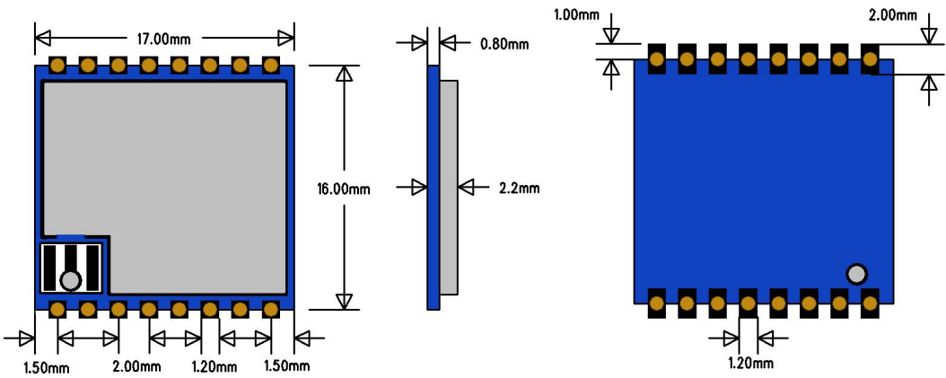
图 3. RC68A 尺寸图
